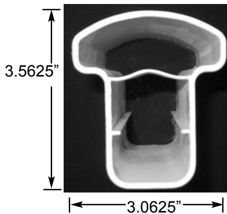
T-Rail
